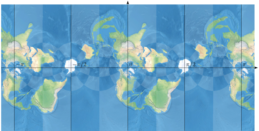
\operatorname{tg} z
