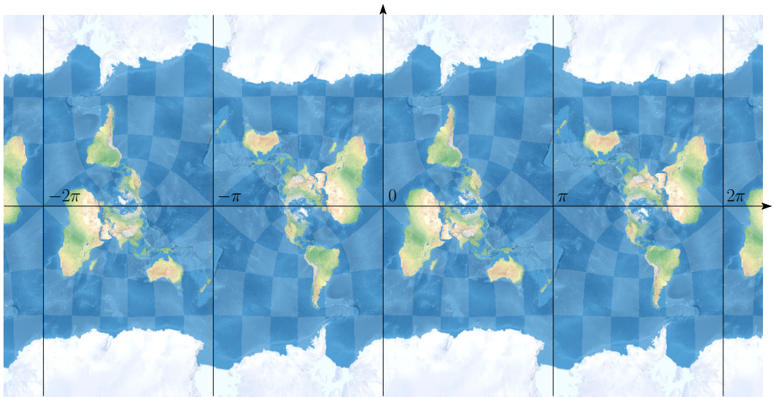
\cos z
