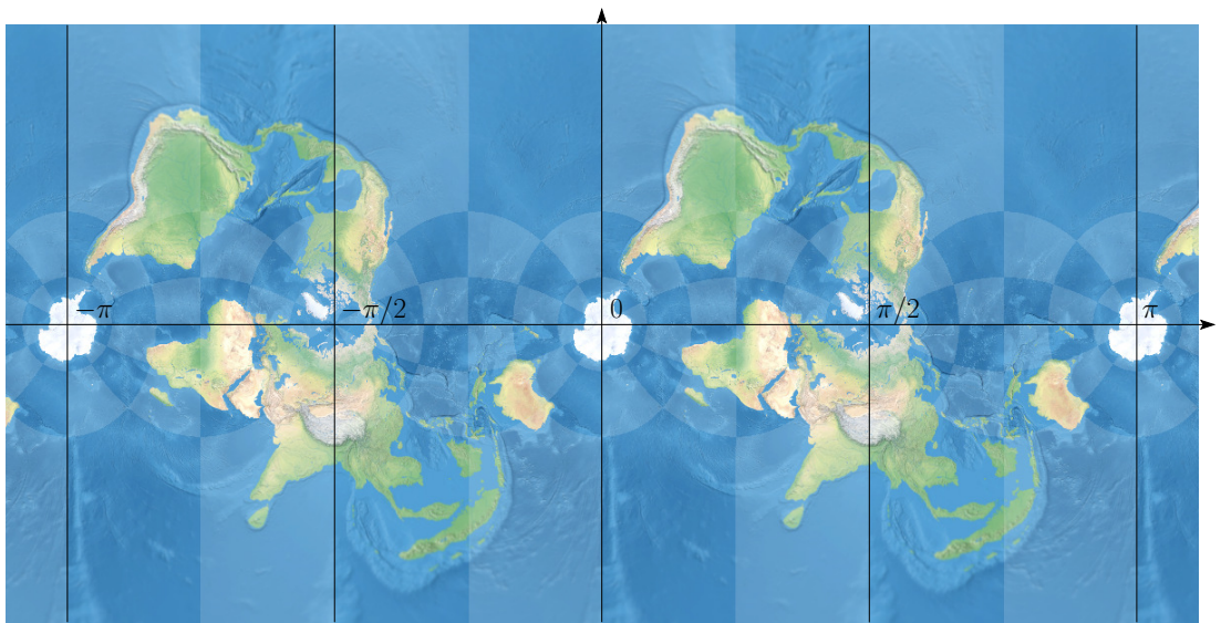
\operatorname{ctg} z
