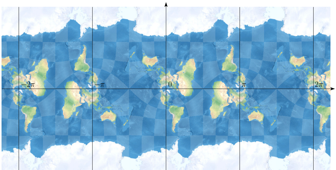
\sin z
