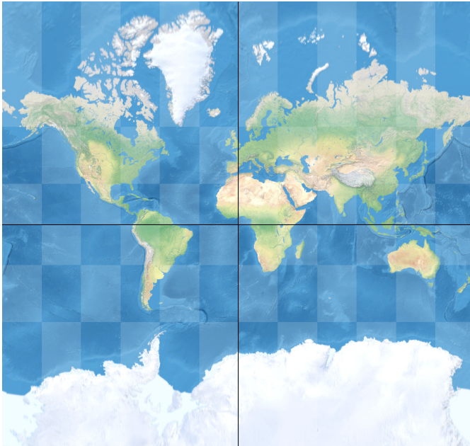
e^{-iz} , Mercator-térkép
