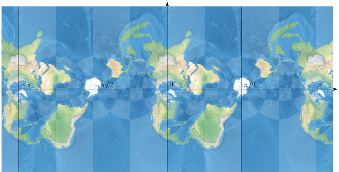
\operatorname{tg} z
